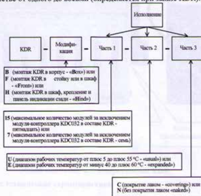
Рисунок 1 – Модификации и исполнения KDR
